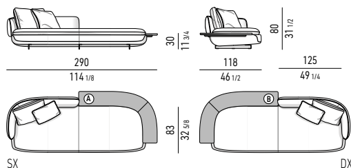
DIVANO CM 290 - SCHIENALE CM 125 CON TOP SOFA CM 290 - BACKREST CM 125 WITH TOP
