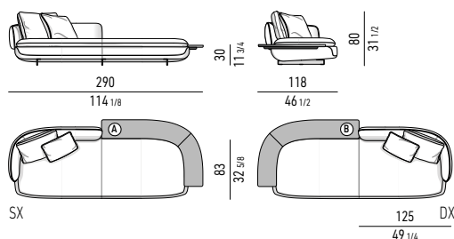
DIVANO CM 290 - SCHIENALE CM 125 CON TOP SOFA CM 290 - BACKREST CM 125 WITH TOP
