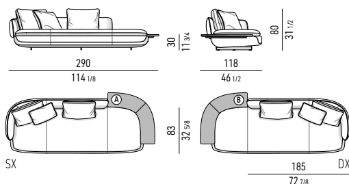
DIVANO CM 290 - SCHIENALE CM 185 CON TOP SOFA CM 290 - BACKREST CM 185 WITH TOP
