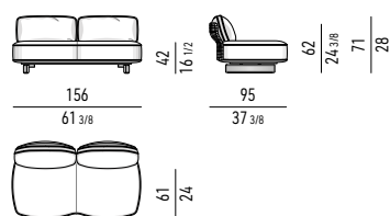
ELEMENTO CENTRALE CM 156X95 CENTRAL ELEMENT CM 156X95
