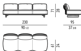
ELEMENTO CENTRALE CM 230X95 CENTRAL ELEMENT CM 230X95
