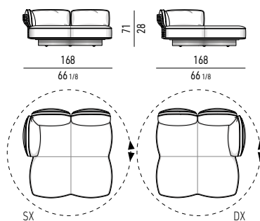
ISOLA CM 168X168 - MOD. B ISLAND CM 168X168 - MOD. B
