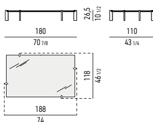
TAVOLINO CM 180X110 H26,5 COFFEE TABLE CM 180X110 H26,5
