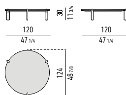
TAVOLINO CM Ø 120 H30 COFFEE TABLE CM Ø 120 H30
