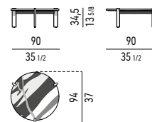
TAVOLINO CM Ø 90 H34,5 COFFEE TABLE CM Ø 90 H34,5
