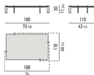
TAVOLINO CM 180X110 H30 COFFEE TABLE CM 180X110 H30
