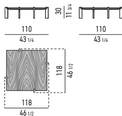
TAVOLINO CM 110X110 H30 COFFEE TABLE CM 110X110 H30
