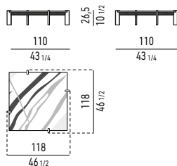
TAVOLINO CM 110X110 H26,5 COFFEE TABLE CM 110X110 H26,5
