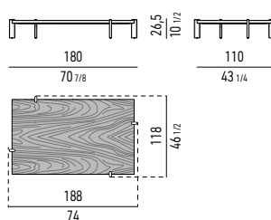
TAVOLINO CM 180X110 H26,5 COFFEE TABLE CM 180X110 H26,5
