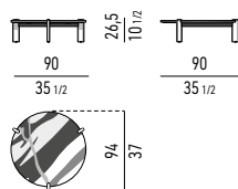
TAVOLINO CM Ø 90 H26,5 COFFEE TABLE CM Ø 90 H26,5
