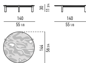
TAVOLINO CM Ø 140 H30 COFFEE TABLE CM Ø 140 H30
