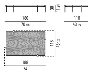
TAVOLINO CM 180X110 H30 COFFEE TABLE CM 180X110 H30
