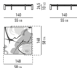
TAVOLINO CM 140X140 H26,5 COFFEE TABLE CM 140X140 H26,5
