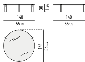
TAVOLINO CM Ø 140 H30 COFFEE TABLE CM Ø 140 H30
