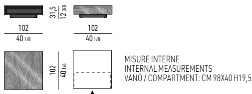
TAVOLINO CM 102X102 H31,5 CON 1 VANO INTERNO COFFEE TABLE CM 102X102 H31,5 WITH 1 INNER COMPARTMENT
