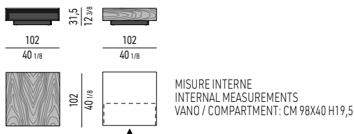
TAVOLINO CM 102X102 H31,5 CON 1 VANO INTERNO COFFEE TABLE CM 102X102 H31,5 WITH 1 INNER COMPARTMENT
