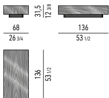
TAVOLINO CM 68X136 H31,5 COFFEE TABLE CM 68X136 H31,5
