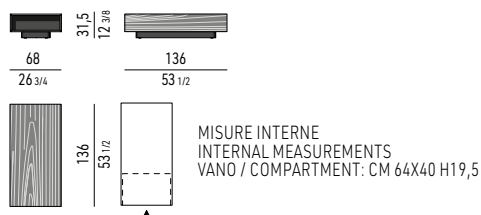
TAVOLINO CM 68X136 H31,5 CON 1 VANO INTERNO COFFEE TABLE CM 68X136 H31,5 WITH 1 INNER COMPARTMENT
