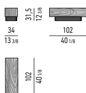
TAVOLINO CM 34X102 H31,5 COFFEE TABLE CM 34X102 H31,5
