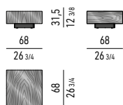
TAVOLINO CM 68X68 H31,5 COFFEE TABLE CM 68X68 H31,5
