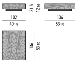
TAVOLINO CM 102X136 H31,5 COFFEE TABLE CM 102X136 H31,5
