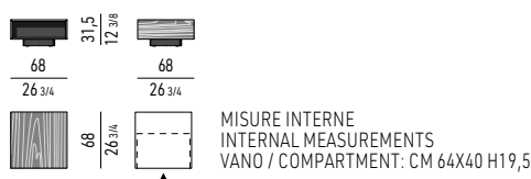
TAVOLINO CM 68X68 H31,5 CON 1 VANO INTERNO COFFEE TABLE CM 68X68 H31,5 WITH 1 INNER COMPARTMENT
