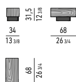
TAVOLINO CM 34X68 H31,5 COFFEE TABLE CM 34X68 H31,5
