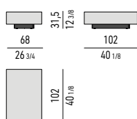
TAVOLINO CM 68X102 H31,5 COFFEE TABLE CM 68X102 H31,5
