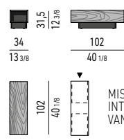
TAVOLINO CM 34X102 H31,5 CON 2 VANI INTERNI COFFEE TABLE CM 34X102 H31,5 WITH 2 INNER COMPARTMENTS
