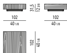
TAVOLINO CM 102X102 H31,5 COFFEE TABLE CM 102X102 H31,5
