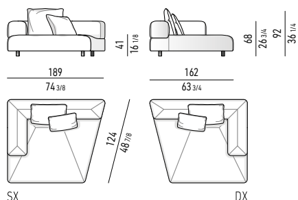
ANGLED CHAISE-LONGUE CM 189X162 - MOD. A ANGLED CHAISE-LONGUE CM 189X162 - MOD. A
