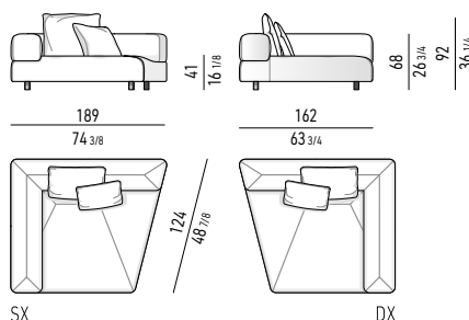
ANGLED CHAISE-LONGUE CM 189X162 - MOD. B ANGLED CHAISE-LONGUE CM 189X162 - MOD. B
